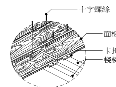
面板交丁處固定詳圖
