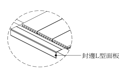
L型收邊條固定詳圖
